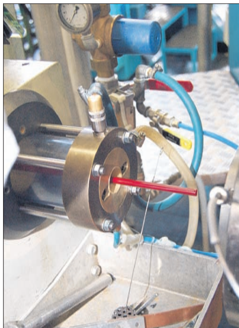
Glattrohr beim Austritt aus der Kalibrierung.
